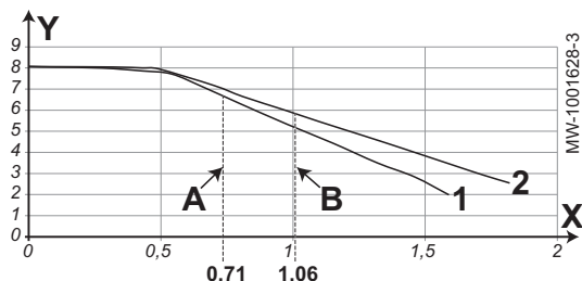
Afb.4 Beschikbare druk
