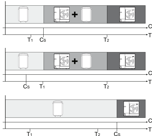
Afb.66 Hybride werkingsprincipe
